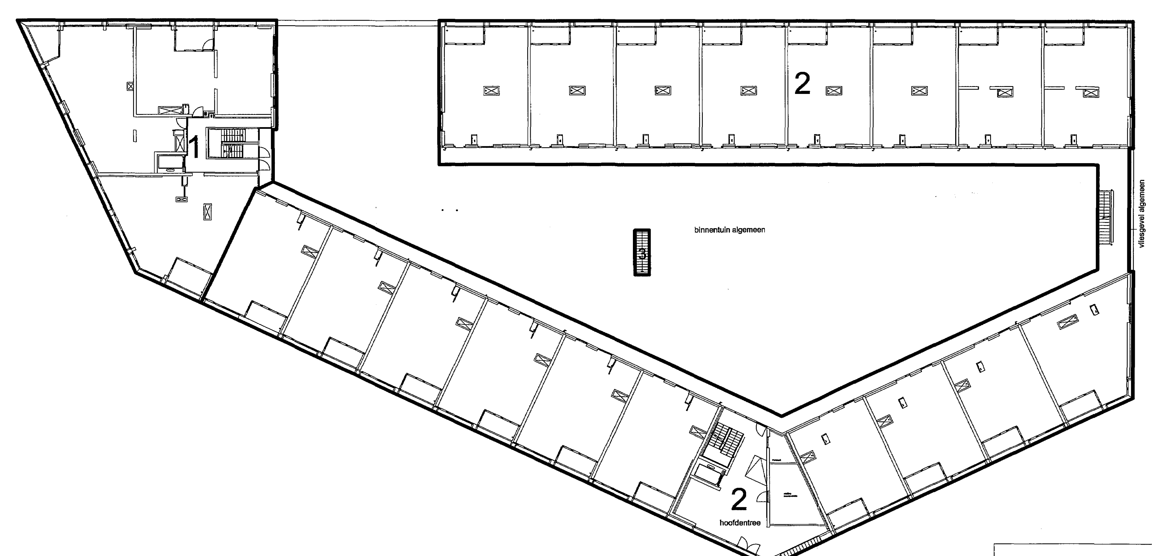
Begane grond schaal 1 : 200
