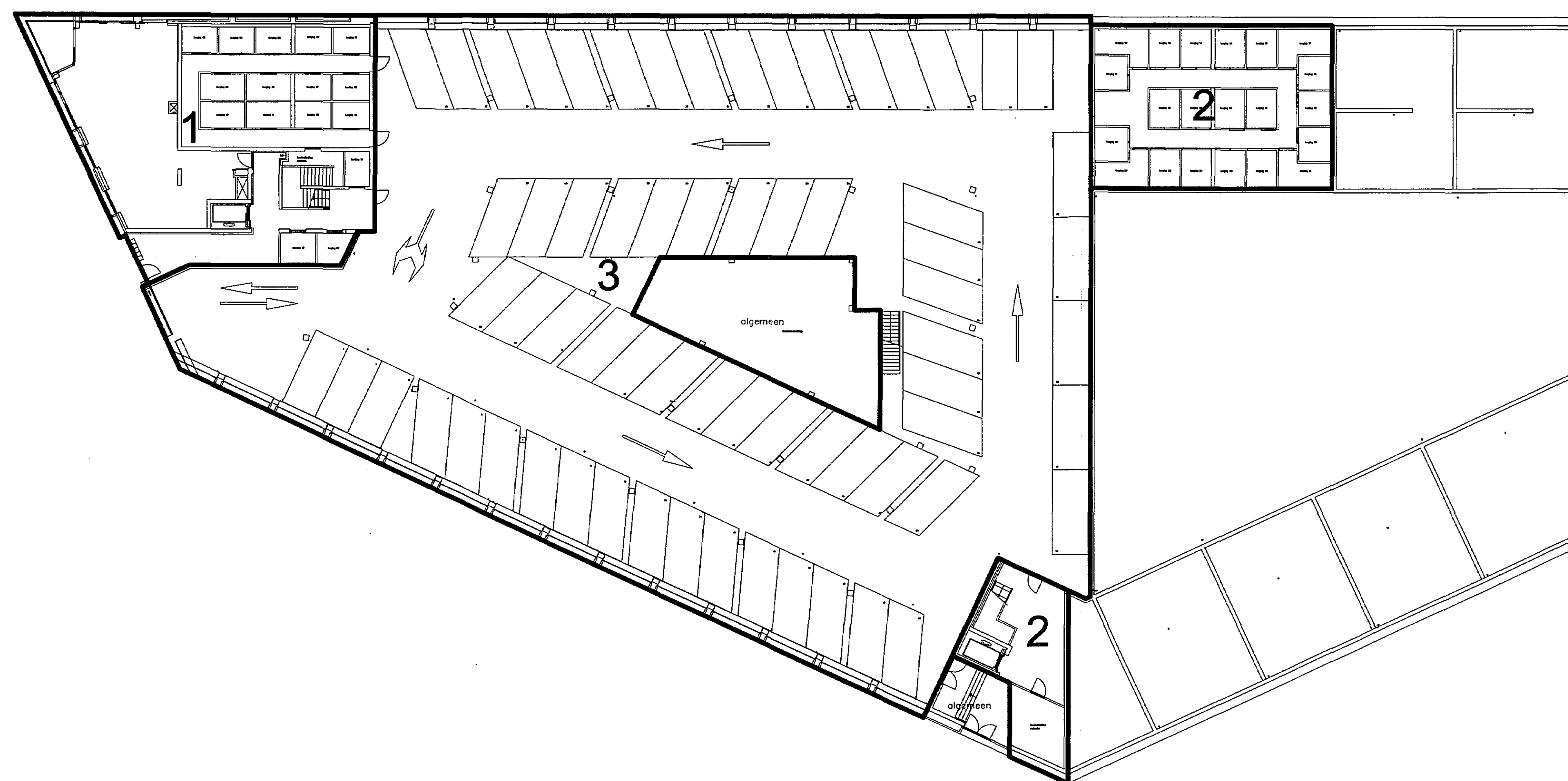
Souterrain schaal 1 : 200
