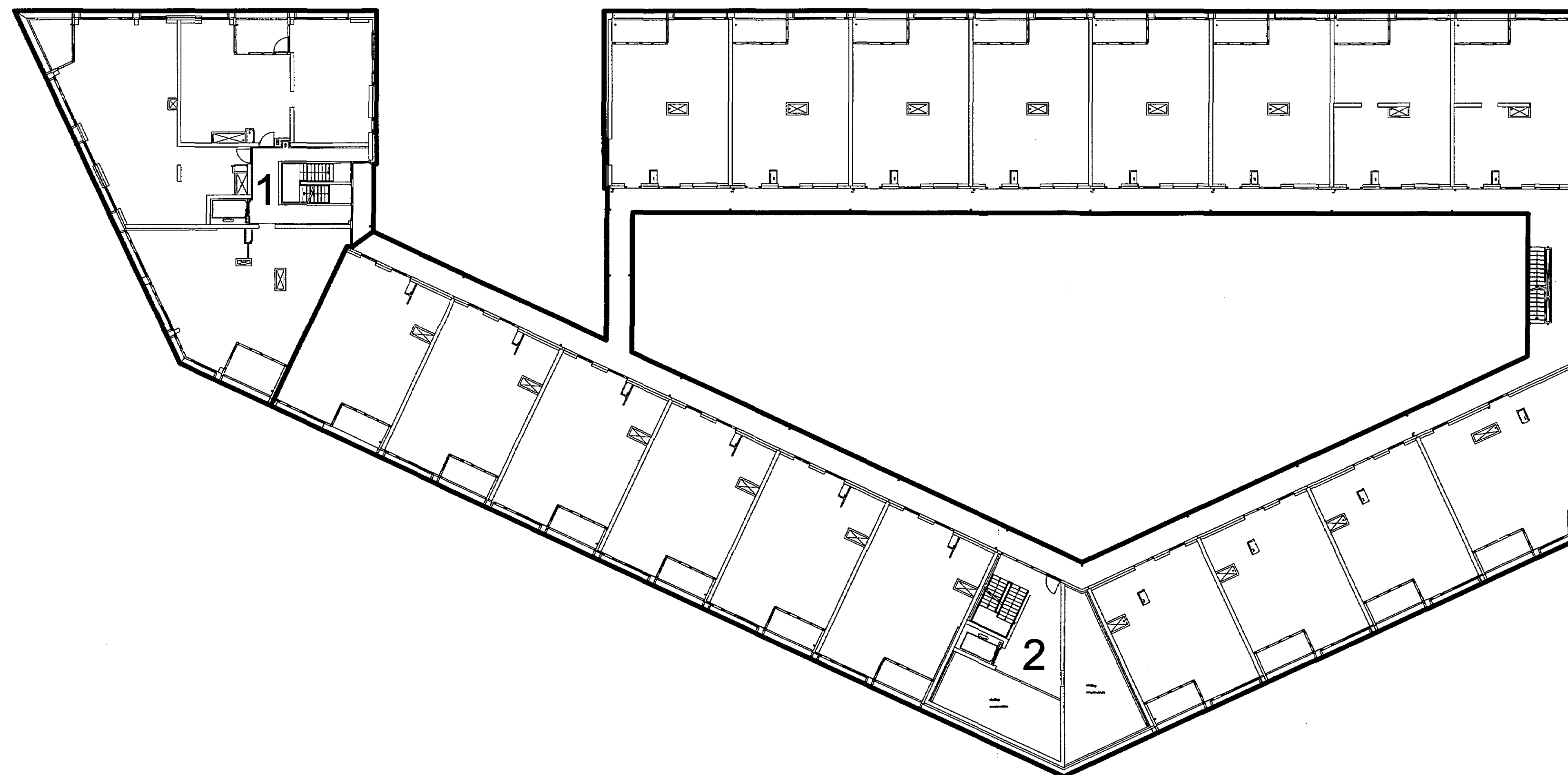
1e verdieping schaal 1 : 200
